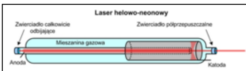
Rysunek 7.3: Schemat budowy lasera He-Ne.
