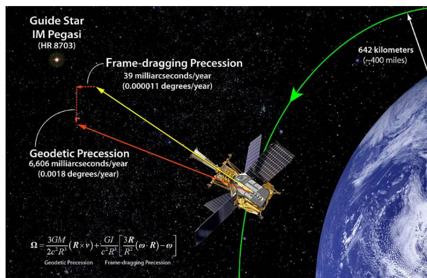
Rysunek 6.14: Schemat doświadczenia “Gravity – probe B” Źródło: Wikipedia
