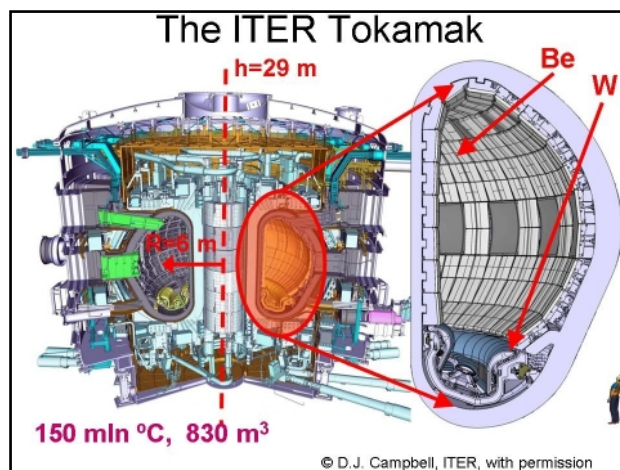
Rysunek 5.6: Schemat budowy reaktora termojądrowego ITER Tokamak w Cadarache w pobliżu Marsylii we Francji z zachowaniem skali. Po prawej stronie na dole stoi dorosły człowiek.
