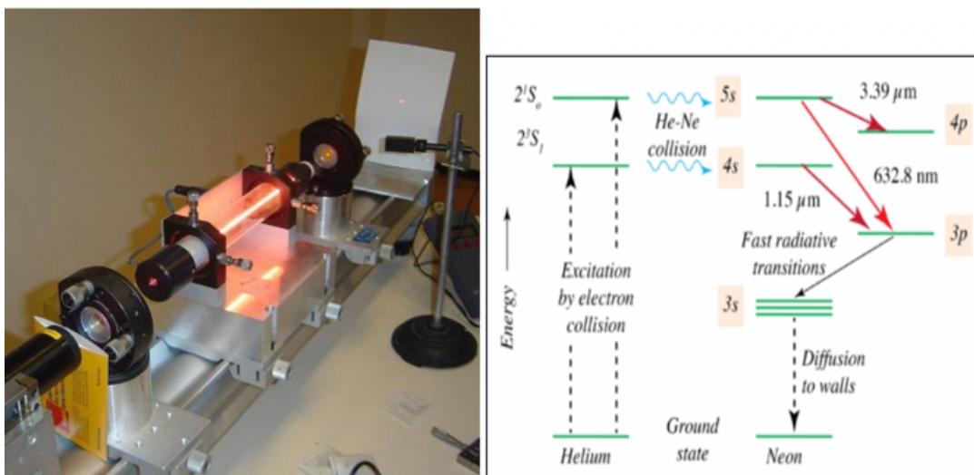
Rysunek 7.2: a) Laser helowo-neonowy emitujący wiązkę światła w zakresie czerwieni i podczerwieni (źródło: Wikipedia ), b) układ poziomów energetycznych w atomach helu i neonu, kluczowe dla działania lasera He-Ne (źródło: Wikipedia )
