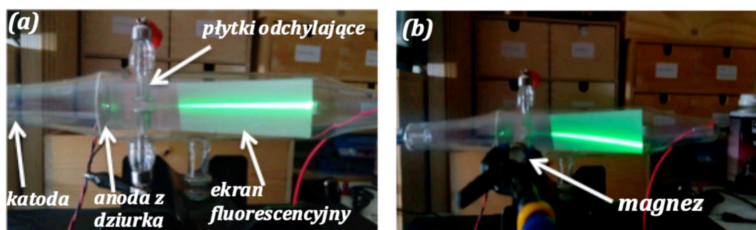
Rysunek 11.8: (a) Promień katodowy rozchodzący się w szklanej rurze z rozrzedzonym gazem. (b) Odchylenie toru promieni katodowych w polu magnetycznym. Źródło: physicsopenlab.org .
