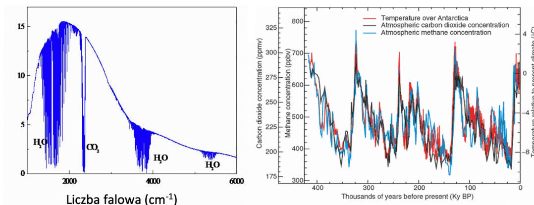
Rysunek 4.4: Mechanizmy efektu cieplarnianego: (lewy rysunek) widmo (natężenie, jednostki względne) promieniowania elektromagnetycznego w temperaturze 290 K ma maksimum w zakresie podczerwieni (długość fali około 9 \mu\text{m} ); N 2 i O 2 w tym zakresie długości fal nie pochłaniają energii, więc atmosfera jest "przezroczysta"; energia jest jednak dobrze pochłaniana przez H 2 O i CO 2 – ich zakresy absorpcji się uzupełniają; CO 2 skutecznie zamyka możliwe okno ucieczki ciepła z Ziemi (pomiar GK); (prawy rysunek) w ciągu ostatnich 400 tys. lat temperatura na Antarktydzie (linia czerwona) i zawartość CO 2 w atmosferze (linia czarna) były ściśle skorelowane (źródło: NOAA).
