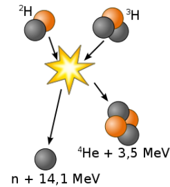
Rysunek 10.9: Schemat syntezy jąder helu ^4\text{He} z jąder deuteru ^2\text{H} i trytu ^3\text{T} , jak w ITER. Źródło: European Nuclear Agency.
