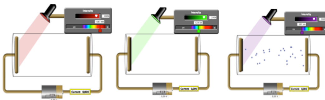
Rysunek 11.5: Efekt fotoelektryczny (wybijanie elektronów z metalu za pomocą światła) pojawia się dla światła o określonym kolorze (tj. długości fali); występowanie efektu fotoelektrycznego nie zależy od natężenia światła. Migawki z symulacji efektu fotoelektrycznego - źródło: phet.colorado.edu .
