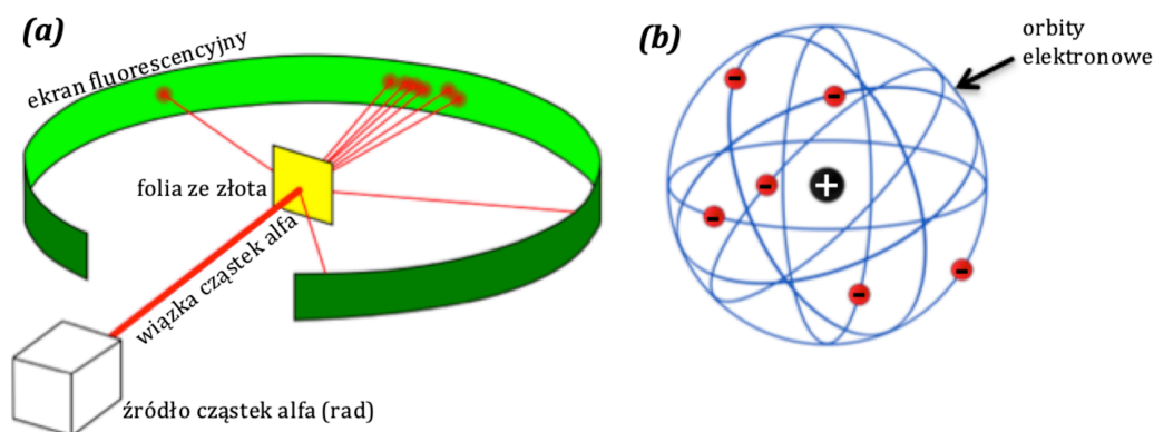
Rysunek 11.10: (a) Schemat eksperymentu Rutherforda – rozpraszanie cząstek alfa na cienkiej folii ze złota. Źródło: large.stanford.edu ; (b) model atomu Rutherforda - źródło: commons.wikimedia.org .
