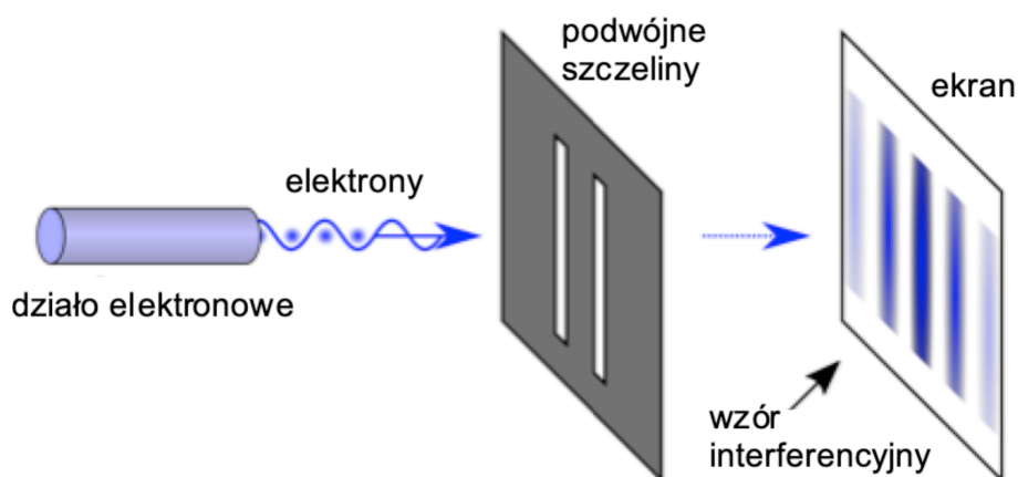
Rysunek 12.4: Schemat eksperymentu Younga (interferencja na podwójnej szczelinie) dla elektronów. Źródło: wikipedia.org .
