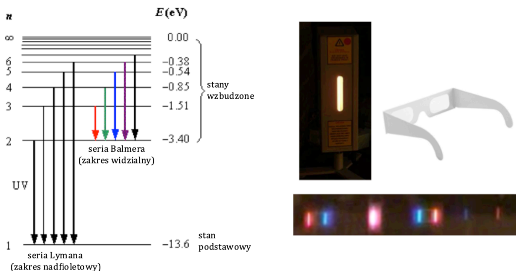
Rysunek 11.11: Układ poziomów energetycznych w atomie wodoru w modelu Bohra; leżąca w zakresie widzialnym seria Balmera odpowiada przeskokom elektronów z orbity o n = 3 na orbitę n = 2 . Rysunek zapożyczony z e-fizyka.info . Serię Balmera można oglądać przy pomocy okularów dyfrakcyjnych i lampy spektralnej z rurką Plückerą wypełnioną wodorem.
