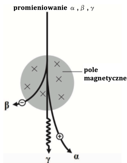
Rysunek 13.2: Promieniowanie \alpha , \beta , \gamma można rozdzielić używając pola magnetycznego. Cząstki \alpha i \beta mają przeciwne ładunki - odchylane są w przeciwne strony, promienie \gamma nie przenoszą ładunku - nie są odchylane.
