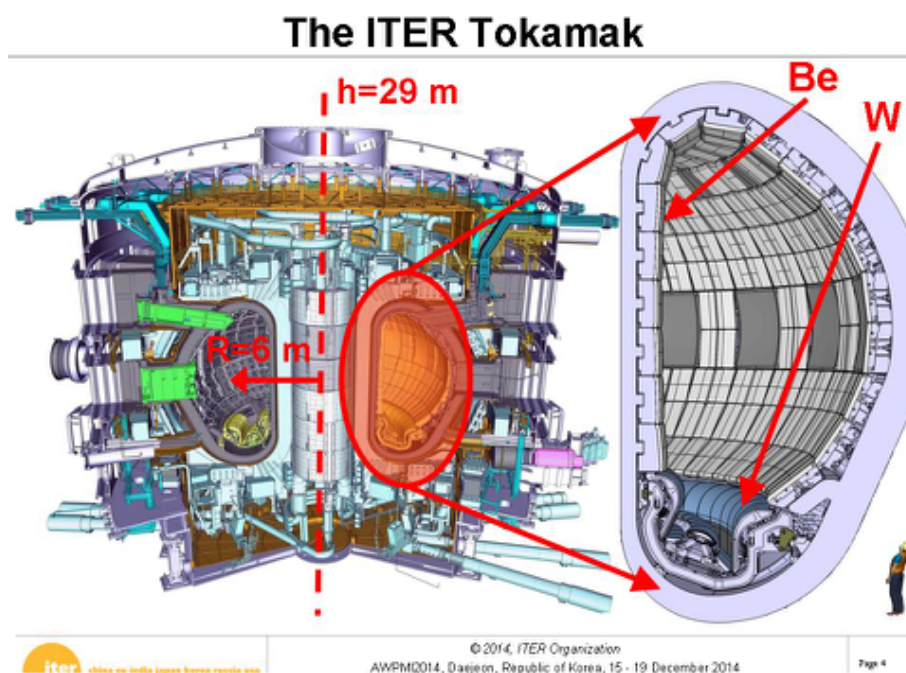
Rysunek 10.10: Schemat reaktora termojądrowego ITER w Cadarache. Credit: dr D. J. Campbell, 2014.
