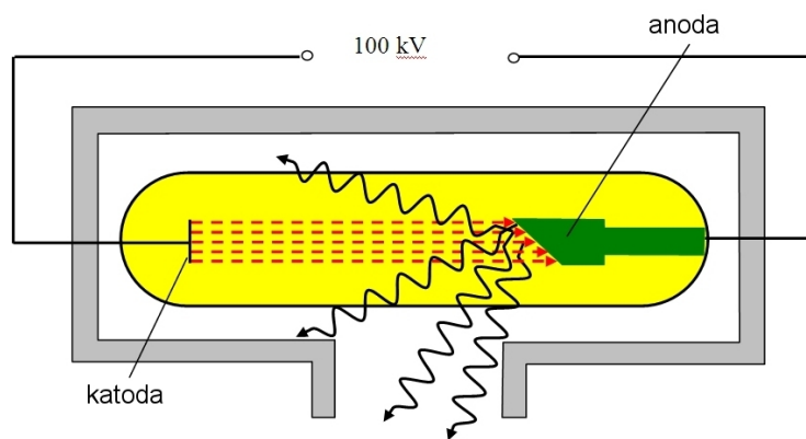
Rysunek 8.2: Schemat lampy rentgenowskiej. Rysunek Eryk Rajch.
