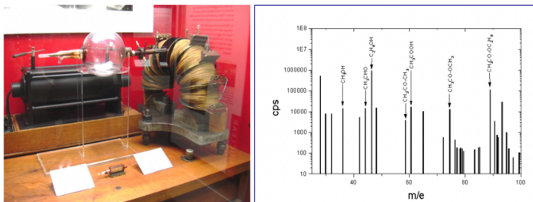
Rysunek 9.6: a) Spektrometr masowy Astona, za pomocą którego stwierdził, m.in., że neon jest mieszaniną atomów o tej samej ilości elektronów ale różnej masie (czyli izotopów). Było to bezpośrednią przesłanką do poszukiwania neutralnego elektrycznie składnika jądra atomowego – neutronu. Muzeum Nauki w Londynie, foto GK, 2001. b) Na powyższym rysunku przedstawione jest widmo masowe powstałe w wyniku jonizacji zapachu świeżych truskawek.
