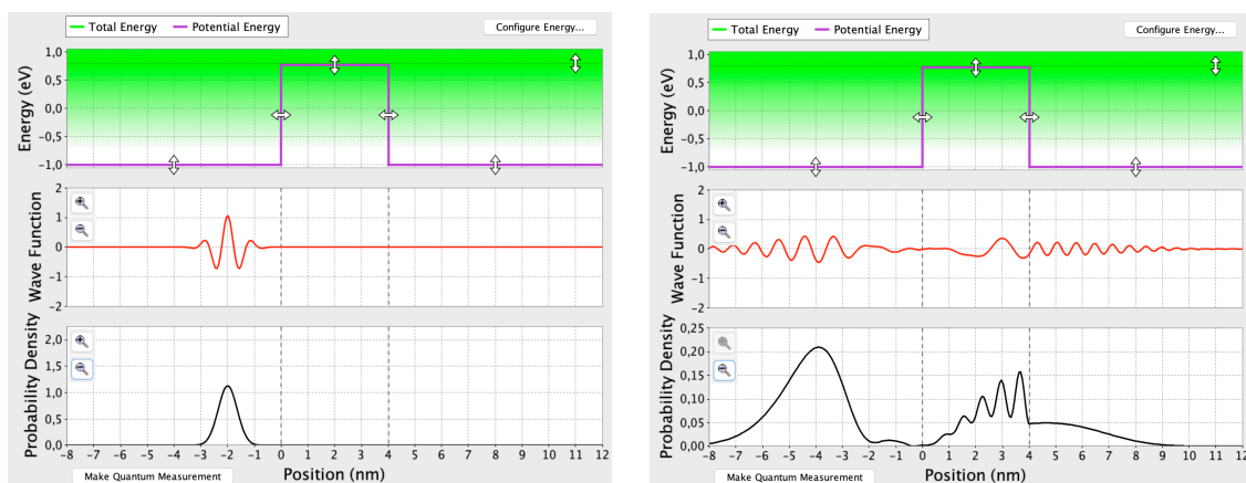
Rysunek 12.7: Symulacja zjawiska tunelowania kwantowego przez prostokątną barierę potencjału w dwóch różnych chwilach czasu. Rysunek lewy : paczka falowa poruszająca się w prawo pada na barierę potencjału o wysokości wyższej niż energia potencjalna cząstki. Pokazana jest tylko część rzeczywista funkcji falowej. Rysunek prawy : Część paczki odbiła się od bariery i porusza się w lewo, druga część tunelowała przez nią i dalej porusza się w prawo. Panel dolny na każdym rysunku przedstawia prawdopodobieństwo znalezienia elektronu wyliczone na podstawie kwadratu funkcji falowej (części rzeczywistej i urojonej). Źródło: Phet.Colorado.edu .
