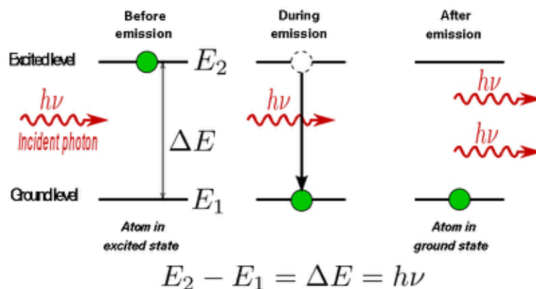
Rysunek 7.1: Schemat emisji wymuszonej dla pojedynczego atomu
