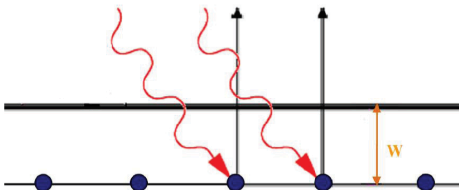
Rysunek 11.6: Schemat efektu fotoelektrycznego: fotony o energii h\nu wybijają elektrony z materiału. Aby elektron mógł opuścić materiał energia fotonu musi być większa niż praca W potrzebna na usunięcie elektronu z ośrodka.
