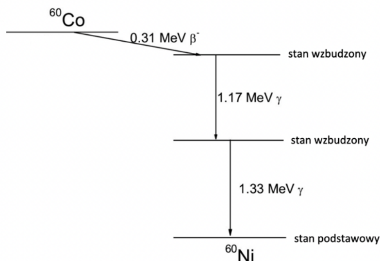
Rysunek 13.6: Schemat rozpadu \beta^- jądra ^{60}_{27}\text{Co} . Procesowi towarzyszy emisja promieniowania o dużej energii kwantów (czyli promieniowanie \gamma ).
