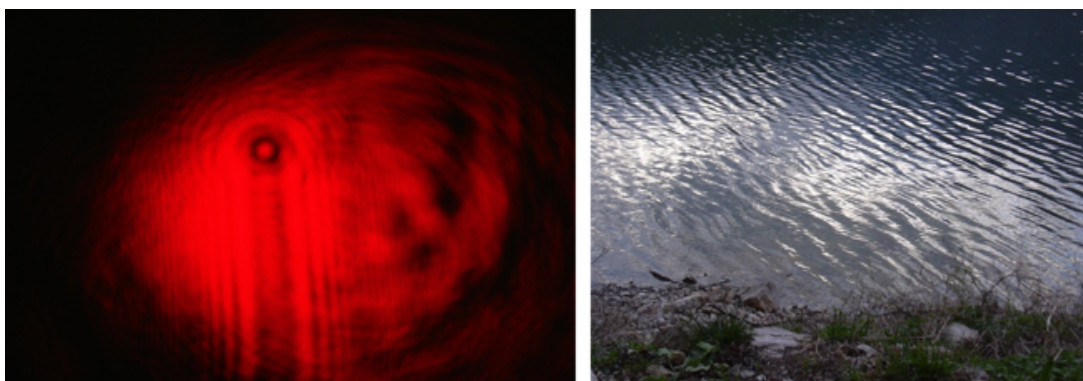
Rysunek 7.7: Ugięcie wiązki światła z lasera na łepku szpilki (foto Krzysztof Służewski) i ugięcie fal na wodzie (foto Maria Karwasz)
