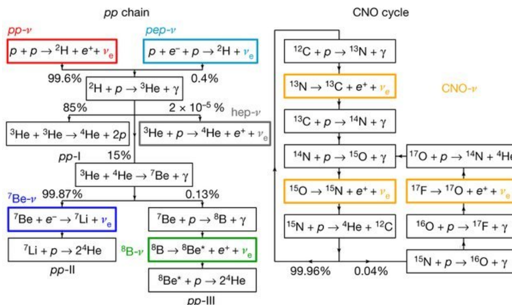
Rysunek 2.11: "Mapa drogowa", czyli kierunki i prawdopodobieństwa zachodzenia reakcji termojądrowych w Słońcu. Reakcje podzielone na cykl protonowy (syntezy helu) i na na cykl syntezy węgla, azotu i tlenu. Oba cykle są połączone wąskim „pomostem” syntezy jądra węgla poprzez stan rezonansowy jądra berylu. Mapa ta ilustruje, że określenie „we wnętrzu Słońca zachodzi synteza cięższych pierwiastków z lżejszych” jest bardzo uproszczone. Źródło: https://www.researchgate.net/publication/328611556_Comprehensive_measurement_of_pp-chain_solar_neutrinos/figures?lo=1
