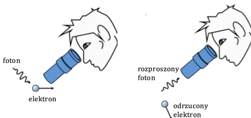
Rysunek 12.9: Pomiar położenia i pędu elektronu za pomocą fotonu. Foton rozprasza się na elektronie w kierunku obserwatora dokonując jednocześnie zaburzenia prędkości badanej cząstki. Rysunek pożyczono z ocw.mit.edu .
