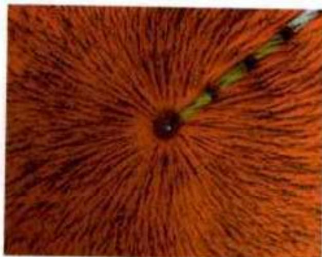
Figura 3. Scoperto il monopolio magnetico?
